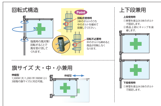
取付図
