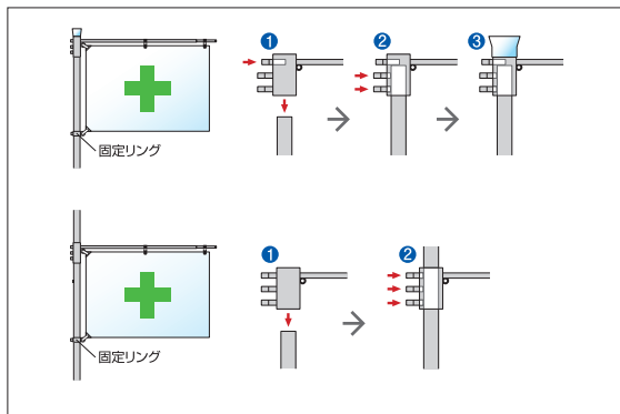
取付図
